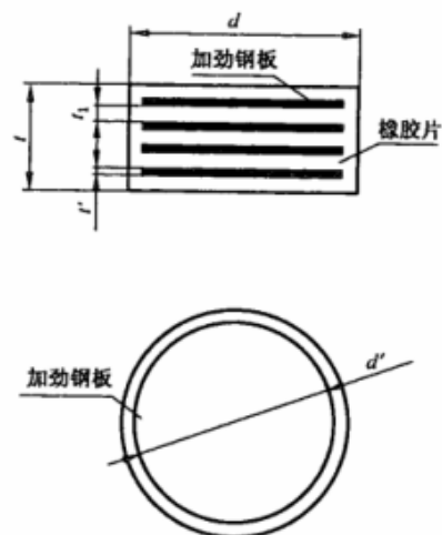
图 2 圆形板式橡胶支座
