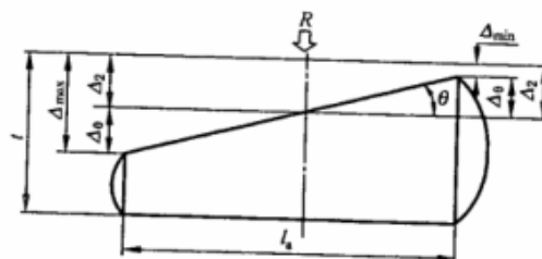
图 A.5 转角计算图
