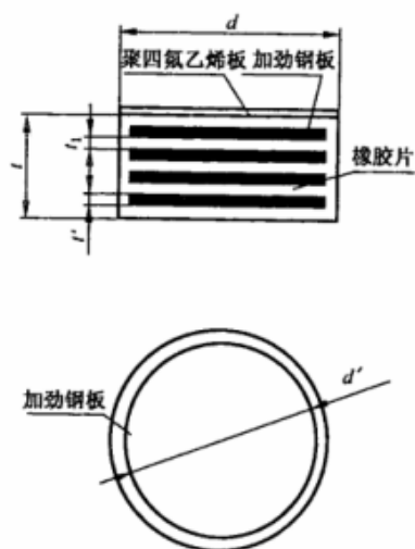
图 4 圆形四氟滑板式橡胶支座
